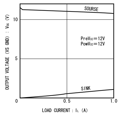
Fig. 8 ch3, 4出力負荷変動
